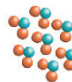
Compuesto formado por átomo de A y B
